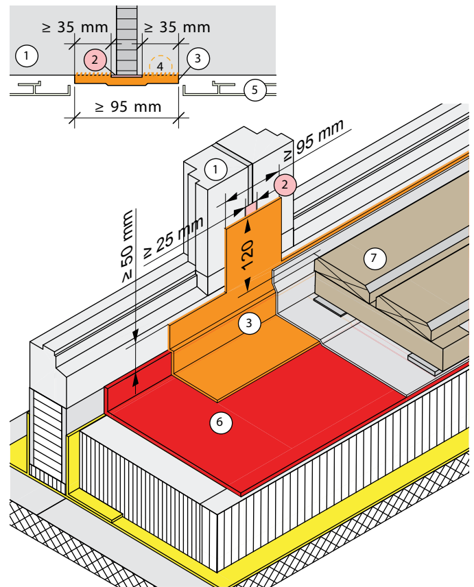
Abb. 49: Elementstoss mit Bewegungsfuge; Rahmen (1), Entkoppelungsband (2), FLK (3), kraftschlüssige Verbindung (4), Metallprofil (5), Abdichtung (6), OK Nutzschicht (7)
